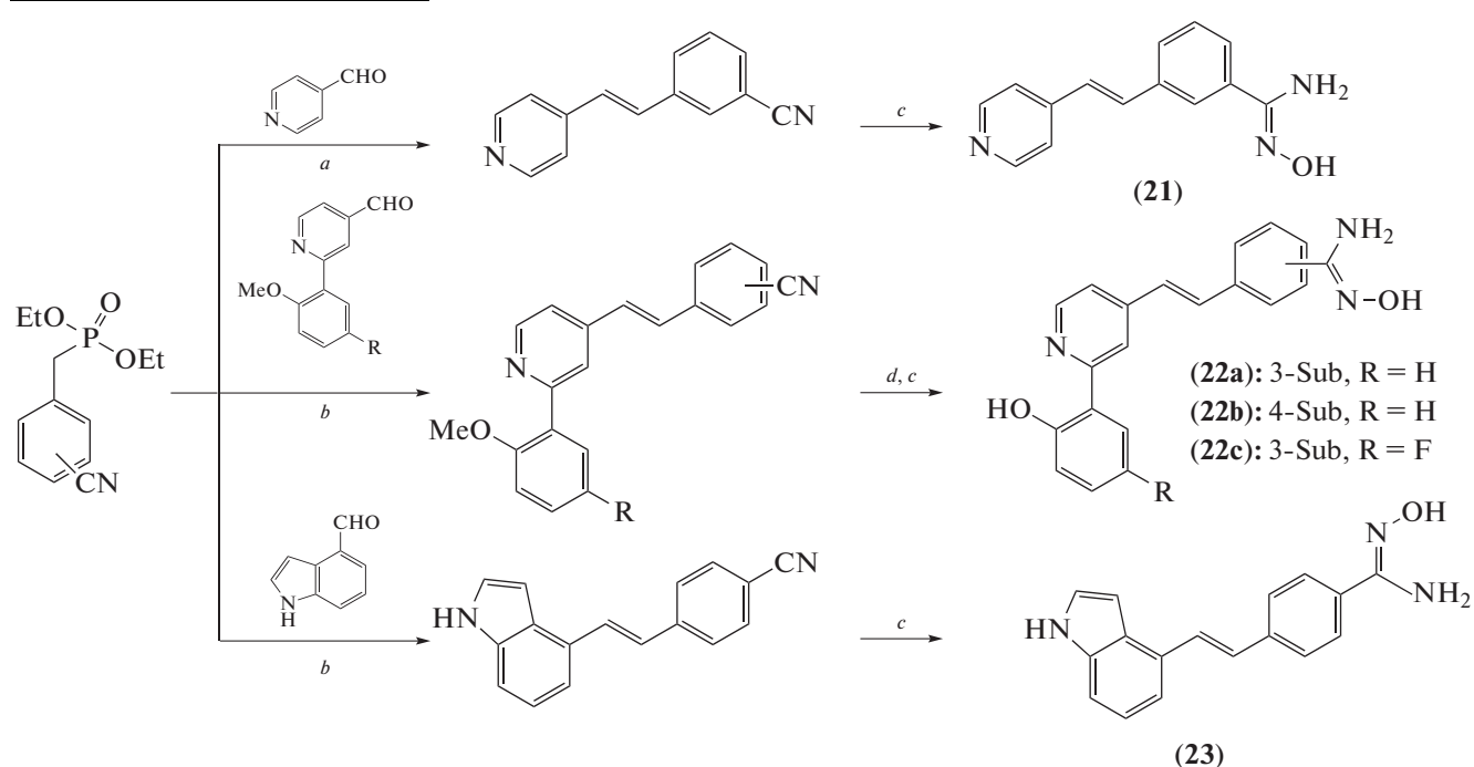
Схема 10. Синтез соединений ( 21–23 ). Реагенты и условия реакций:
